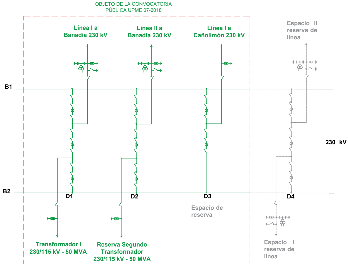
Figura 3. Diagrama Unifilar Subestación La Paz 230 kV (Prepublicación)
