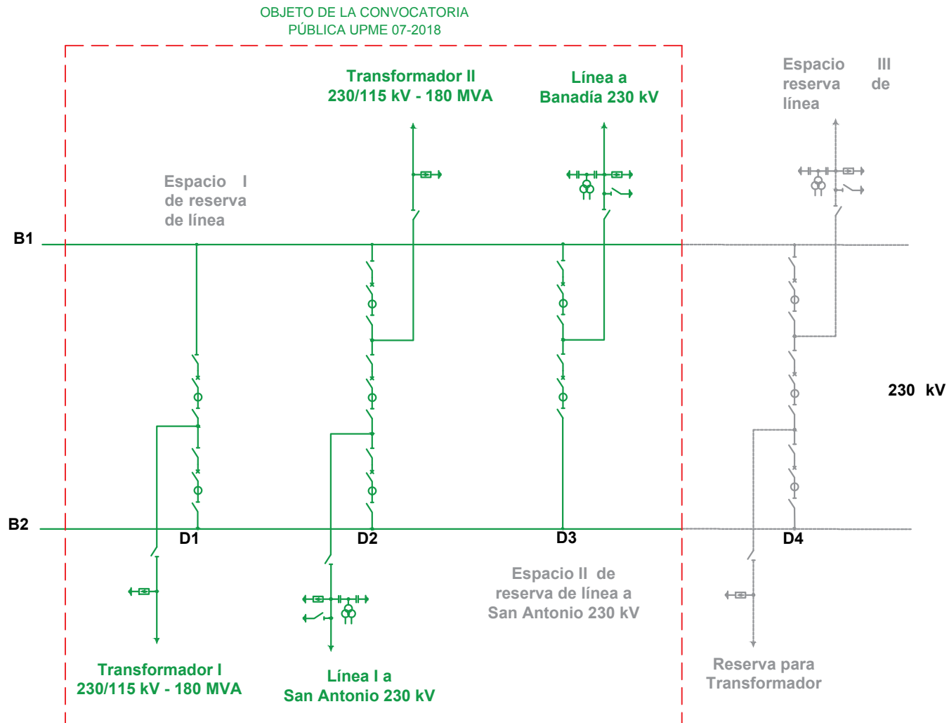
Figura 2. Diagrama Unifilar Subestación Alcaravan 230 kV (Prepublicación)
