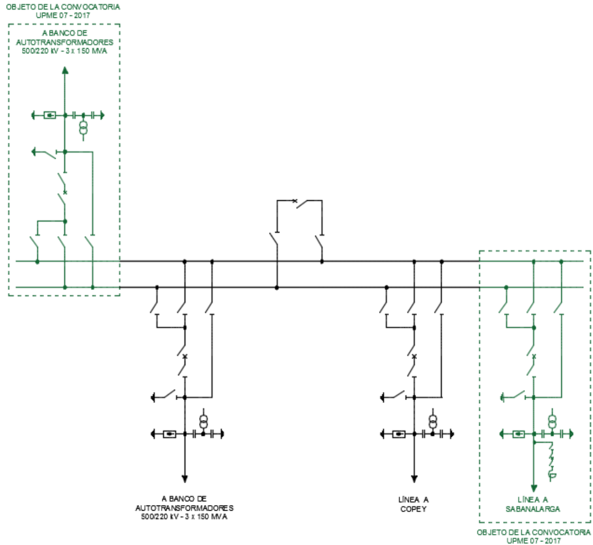
FIGURA 3. SUBESTACIÓN BOLÍVAR 500 kV (PREPUBLICACIÓN)
