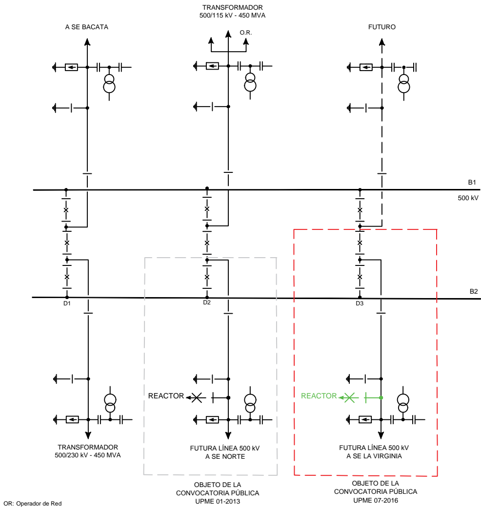
FIGURA 2 ESQUEMA UNIFILAR SUBESTACIÓN NUEVA ESPERANZA 500 kV
