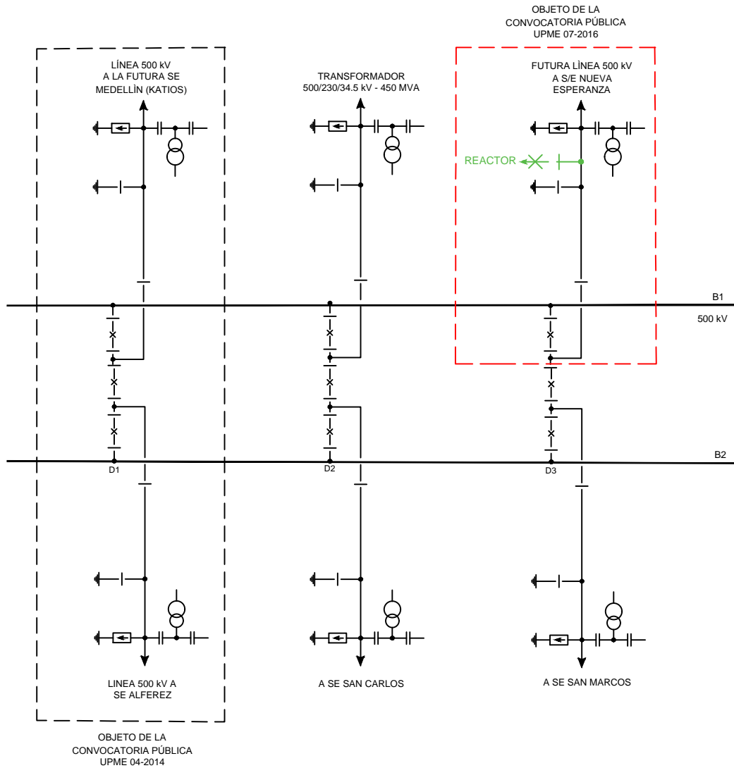
FIGURA 1 ESQUEMA UNIFILAR SUBESTACIÓN LA VIRGINIA 500 kV
