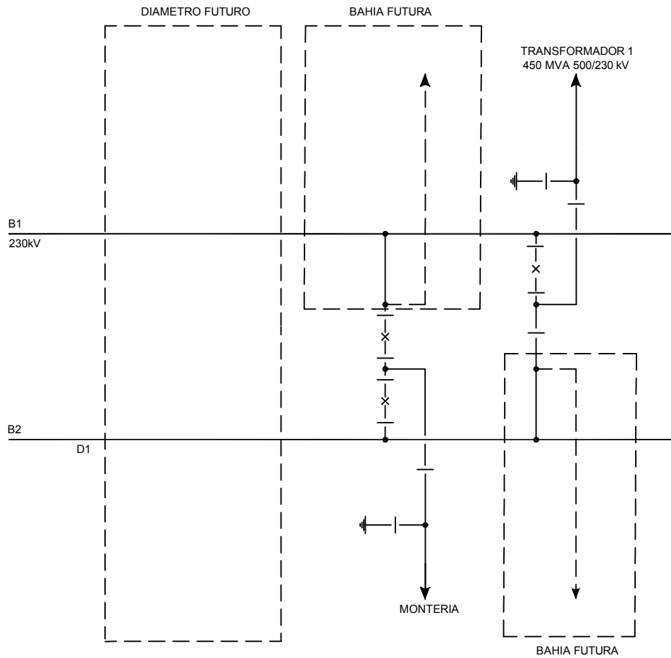
FIGURA 4 ESQUEMA UNIFILAR SUBESTACIÓN CHINU 230kV
