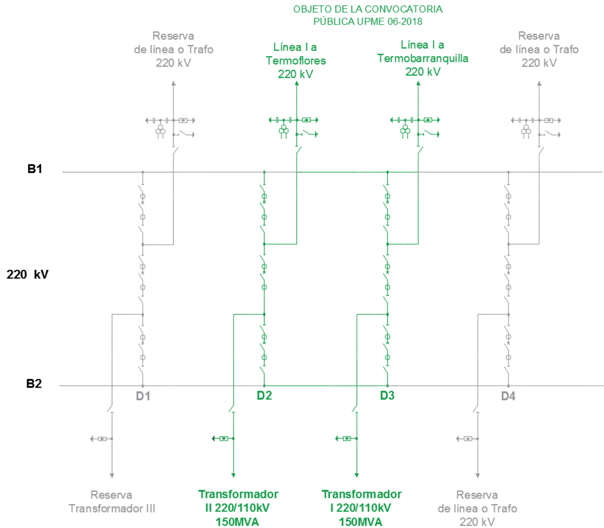
Figura 2 - Diagrama Unifilar Subestación El Rio 220 kV
