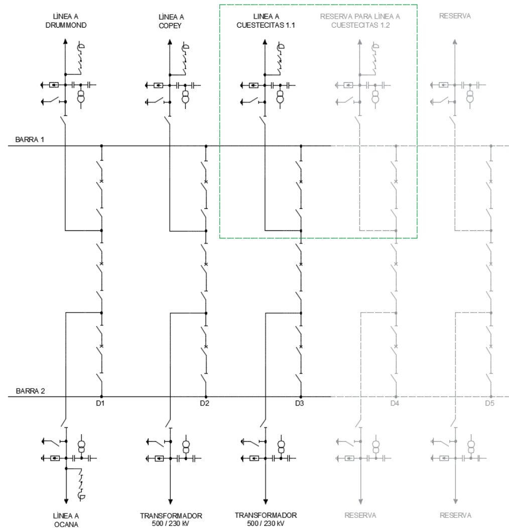
FIGURA 4 SUBESTACIÓN LA LOMA 500 kV
