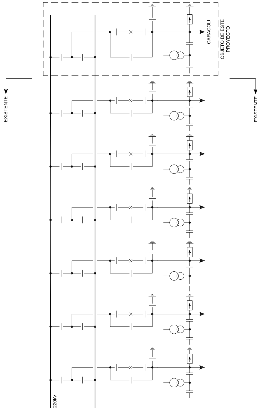
FIGURA 3 ESQUEMA UNIFILAR AMPLIACIÓN DE SUBESTACIÓN FLORES 220kV
