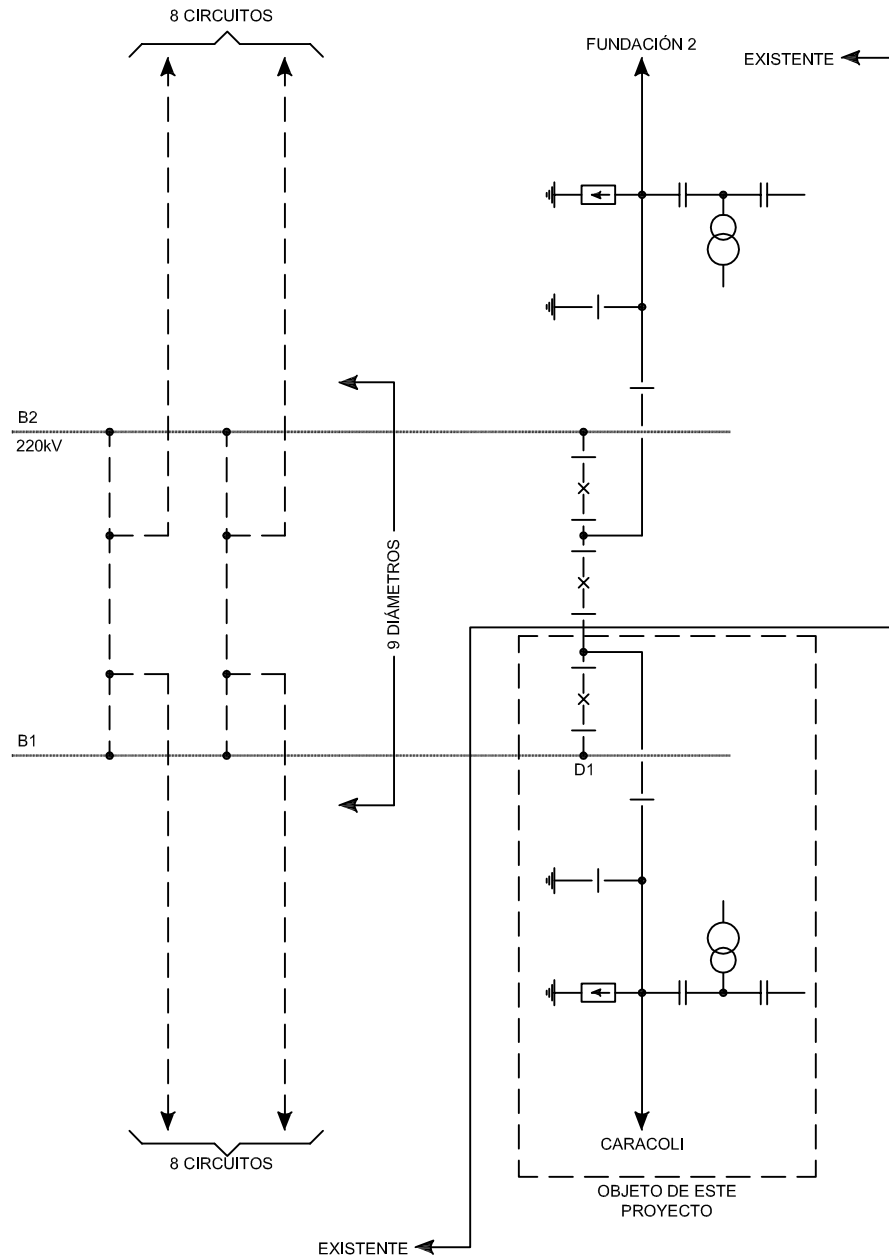
FIGURA 5 ESQUEMA UNIFILAR AMPLIACIÓN SUBESTACIÓN SABANALARGA 220kV
