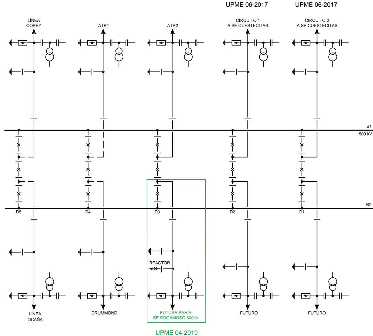
Figura 2. Diagrama Unifilar La Loma 500 kV (Prepublicación)
