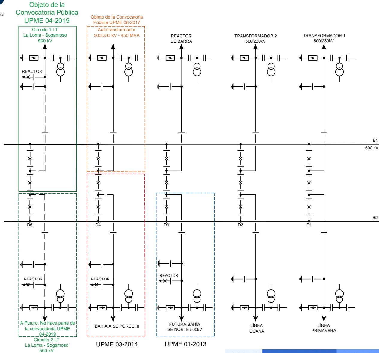
Figura 3. Diagrama Unifilar Sogamoso 500 kV
