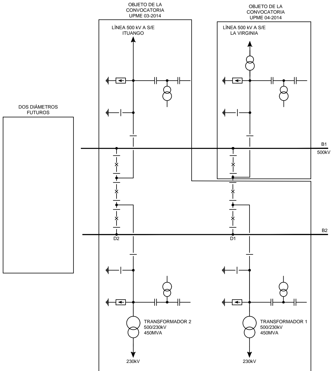
FIGURA 7 ESQUEMA UNIFILAR SUBESTACIÓN MEDELLIN 500kV
