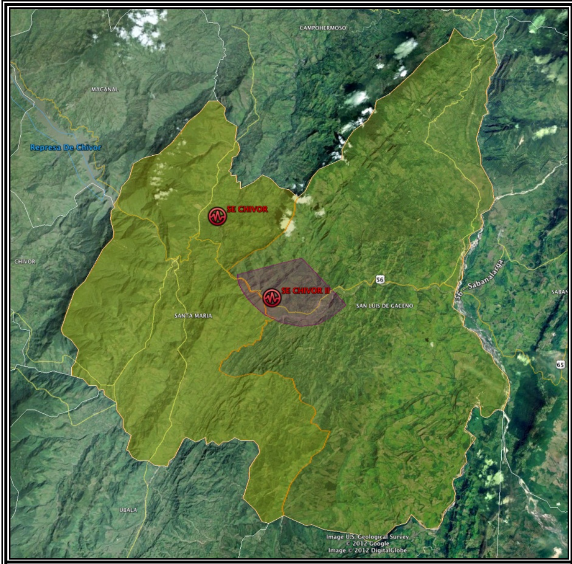
Figura 3 Área identificada por UPME a nivel de referencia para la ubicación de la Subestación Chivor II
