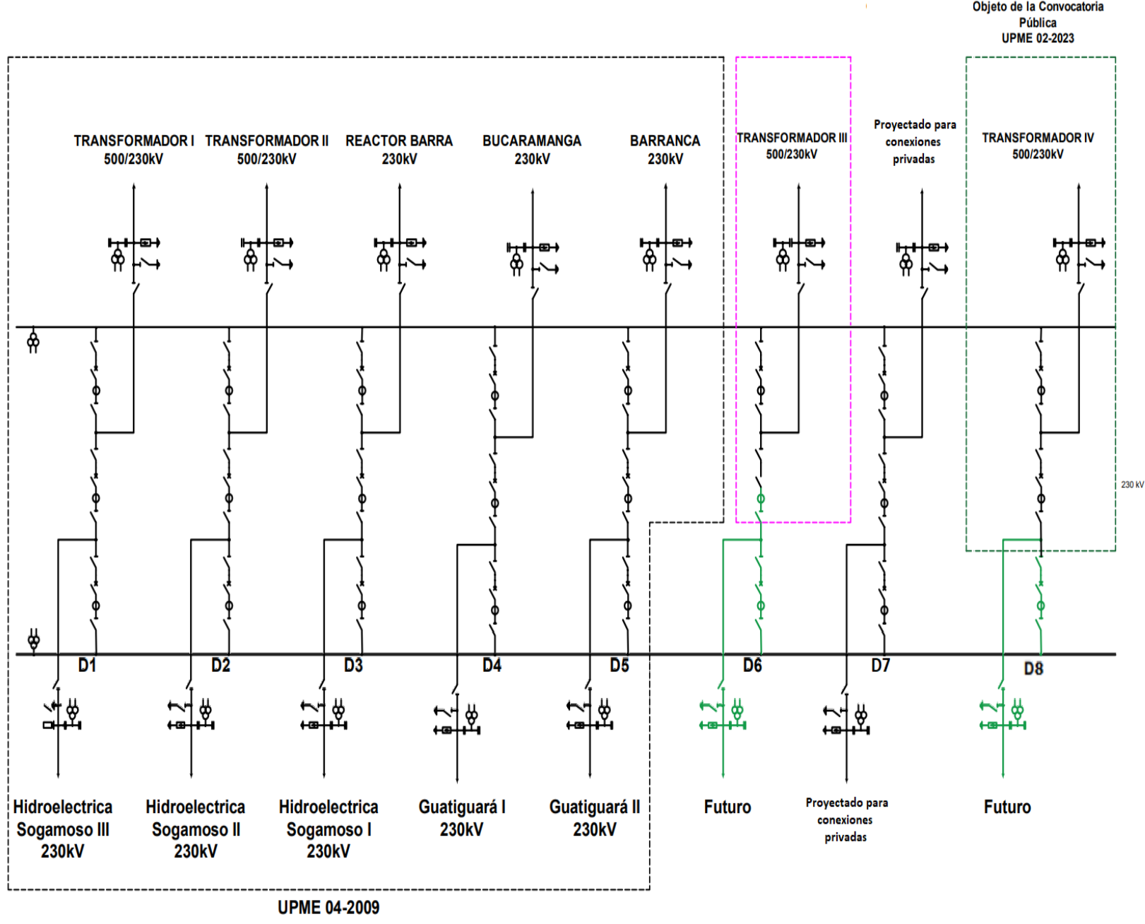
FIGURA 2 ESQUEMA UNIFILAR SUBESTACIÓN SOGAMOSO 230kV
