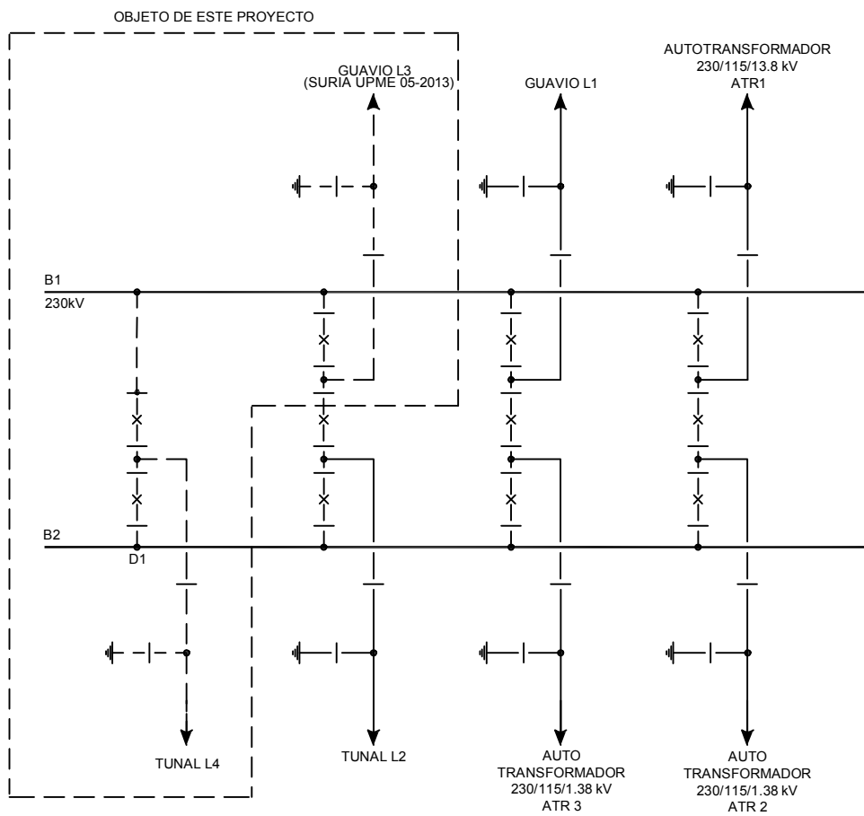
FIGURA 1 ESQUEMA UNIFILAR SUBESTACIÓN REFORMA 230kV CONVOCATORIA UPME 02-2014
