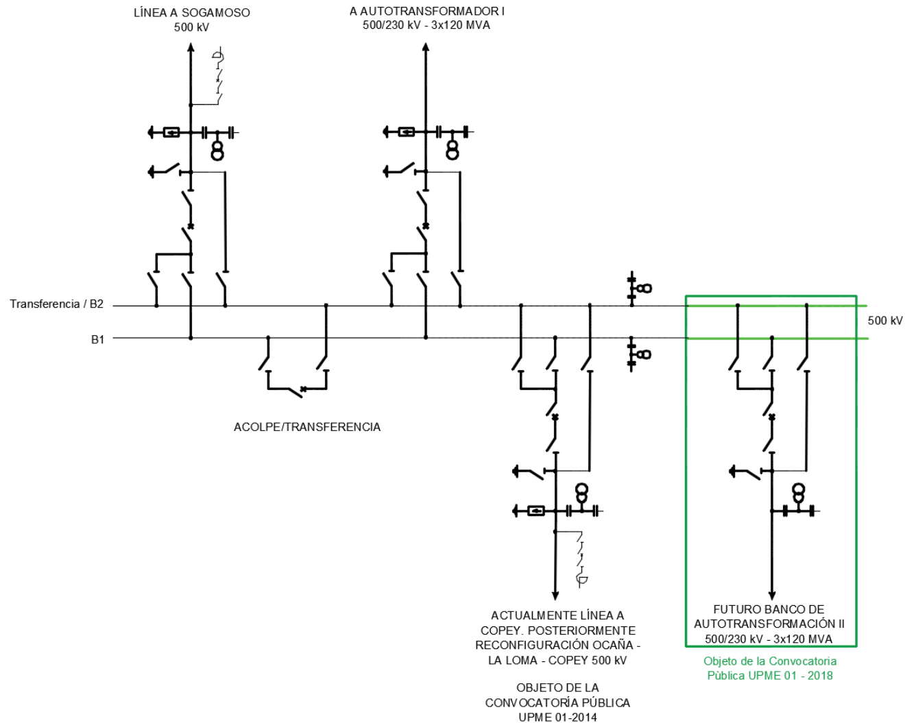
Figura 1 - Diagrama Unifilar Subestación Ocaña 500 kV
