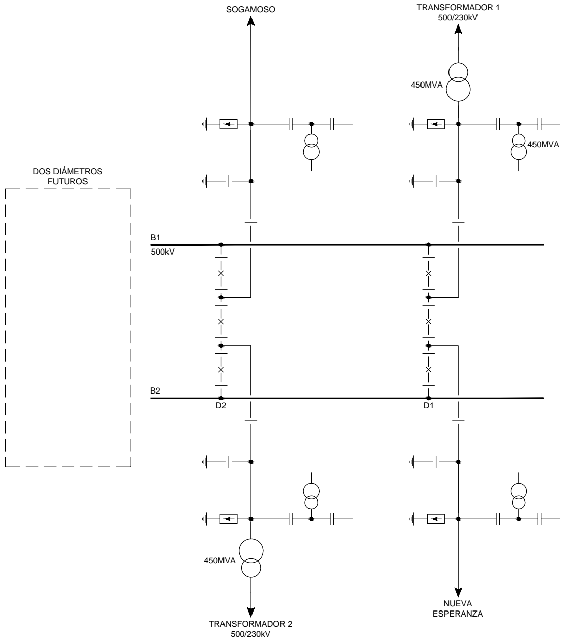
FIGURA 4 ESQUEMA UNIFILAR SUBESTACIÓN NORTE 500kV
