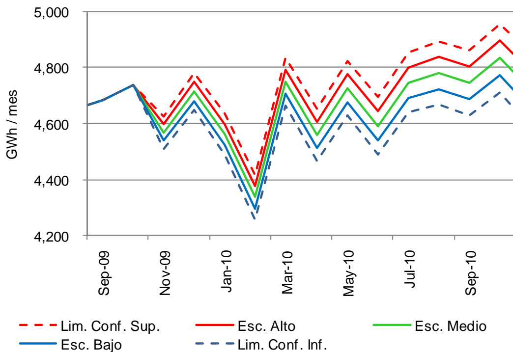
Gráfica C - 1 Escenarios de proyección mensual de demanda de energía eléctrica y límites de confianza, 2009-2010.
