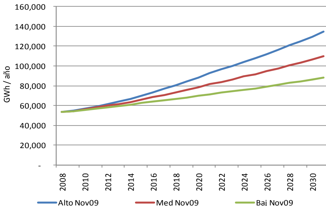
Gráfica 3.5. Banda de proyección de demanda nacional de energía eléctrica 2009-2031.
