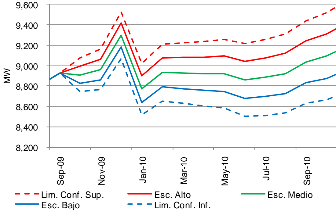
Gráfica C - 2 Escenarios de proyección mensual de potencia eléctrica máxima y límites de confianza, 2009-2010.
