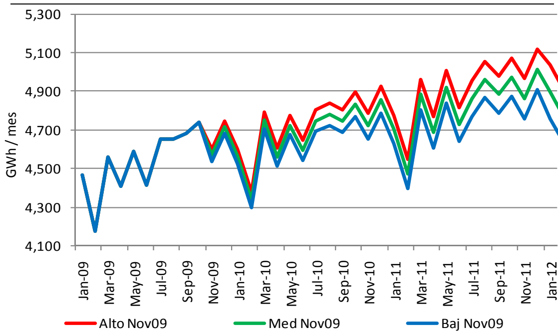
Gráfica 3.3. Banda de proyección de demanda nacional de energía eléctrica 2009-2011.
