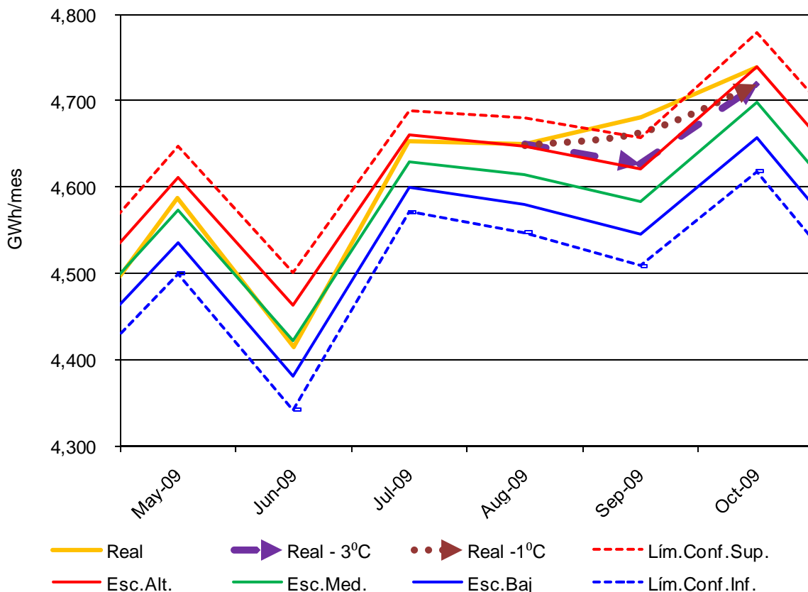
Gráfica D - 3 Efectos de las altas temperaturas sobre la demanda de energía eléctrica en los meses de septiembre y octubre de 2009.
