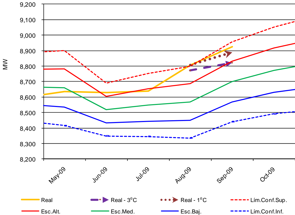
Gráfica 2.4. Desviación del pronóstico de potencia, último año.
