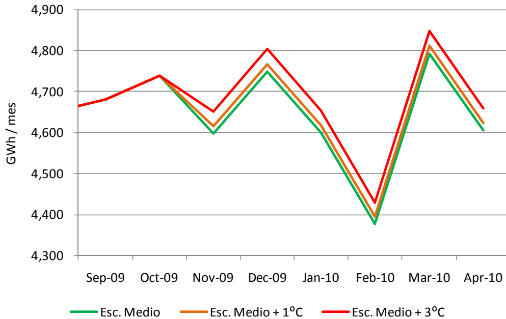
Gráfica D - 4 Efectos de las altas temperaturas sobre la proyección de demanda de energía eléctrica en los próximos meses.
