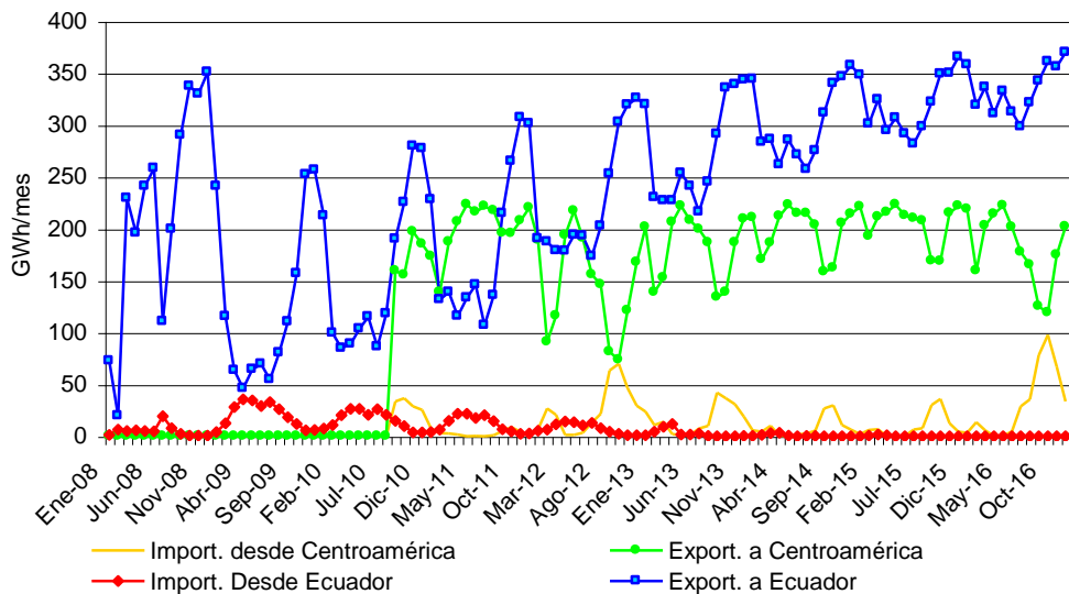
Gráfica E - 1 Proyección de exportaciones e importaciones de energía eléctrica de Colombia
