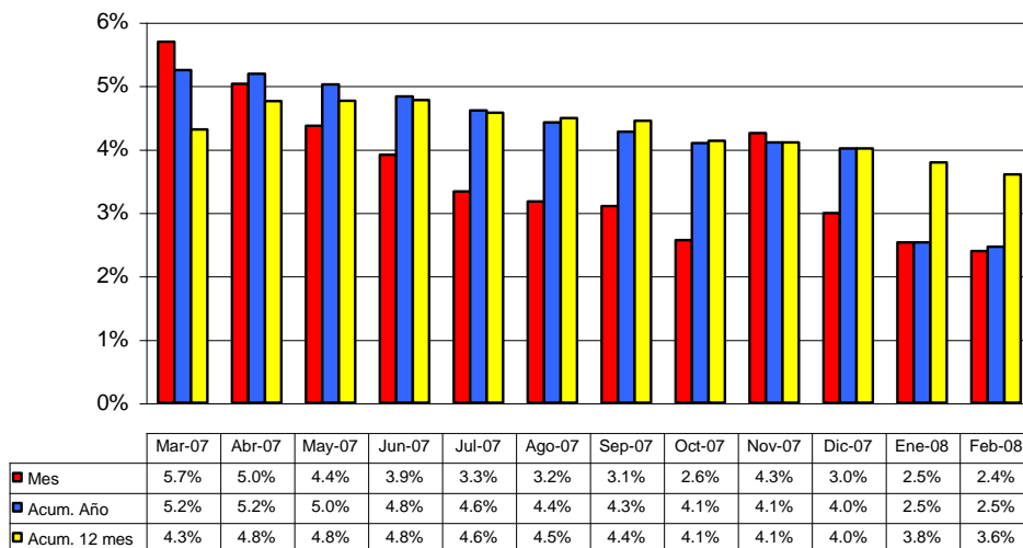
Gráfica 3.1 Crecimiento mensual de la demanda de energía eléctrica, último año
