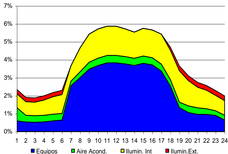
b)- Curva de carga sector terciario Escenario 3
